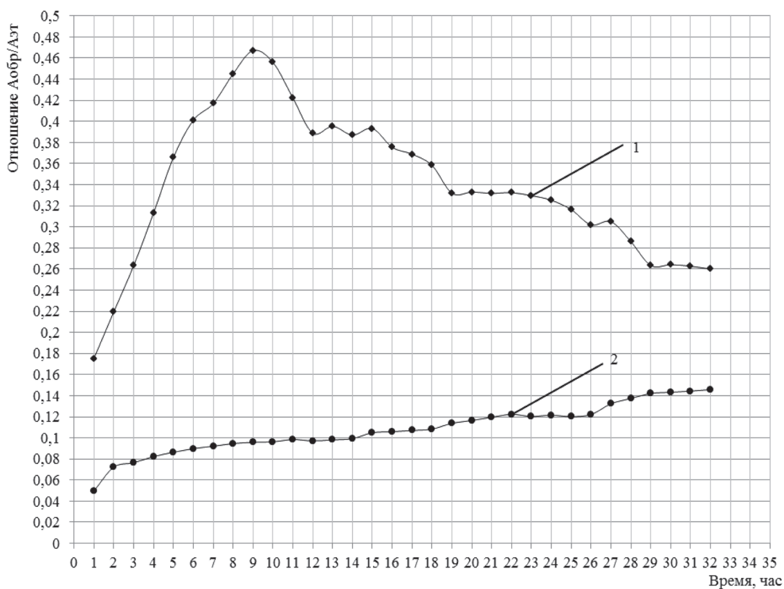
Рис. 3. Кинетика активности системы отверждения БК в присутствии П-23 в зависимости от температуры: 1 – при 80 °С, 2 – при 55 °С
