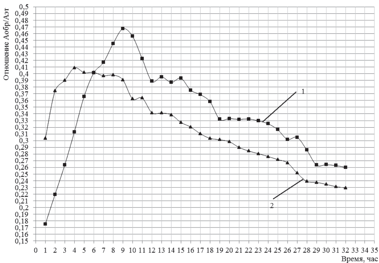
Рис. 2. Кинетика активности системы отверждения БК в присутствии П-23 и без него при 80 °С: 1 – 1,8 %; 2 – без П-23
