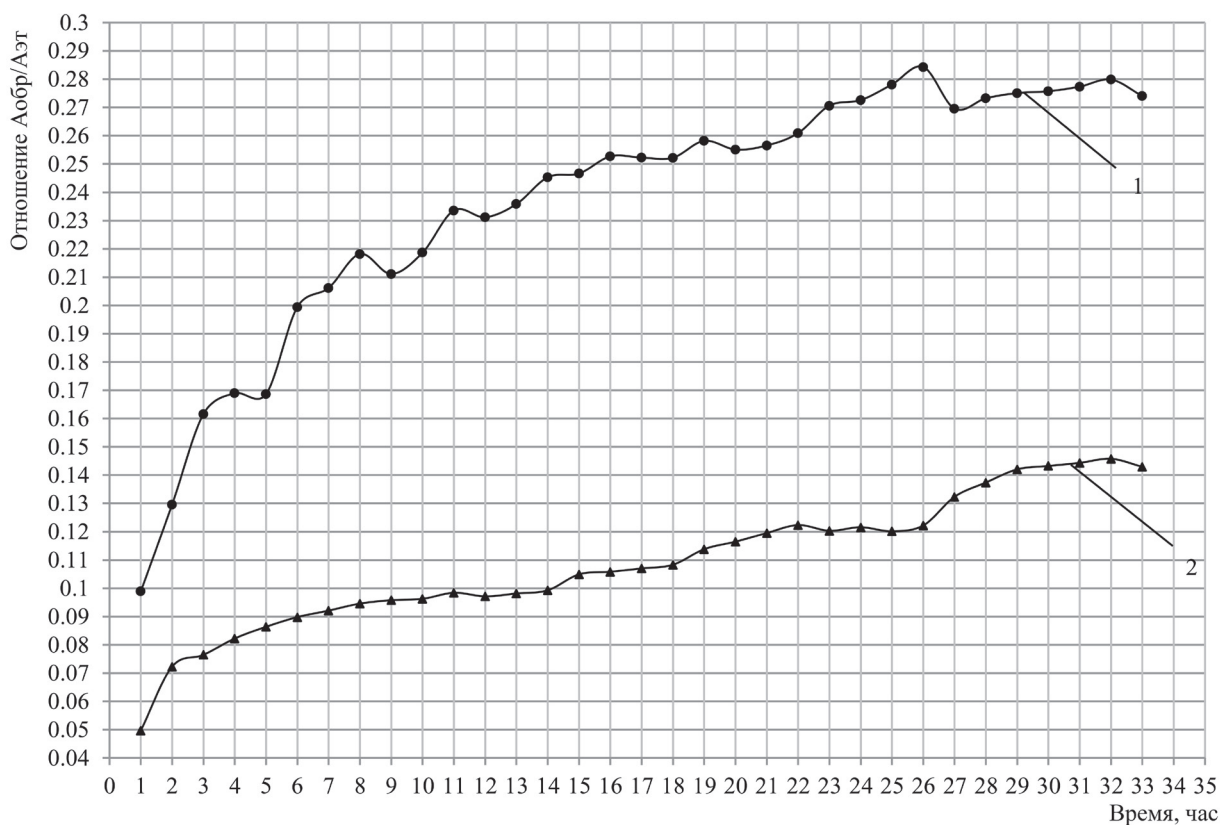
Рис. 1. Кинетика активности системы отверждения БК в присутствии П-23 и без него при 55 °С: 1 – без П-23; 2 – 1,8 %
