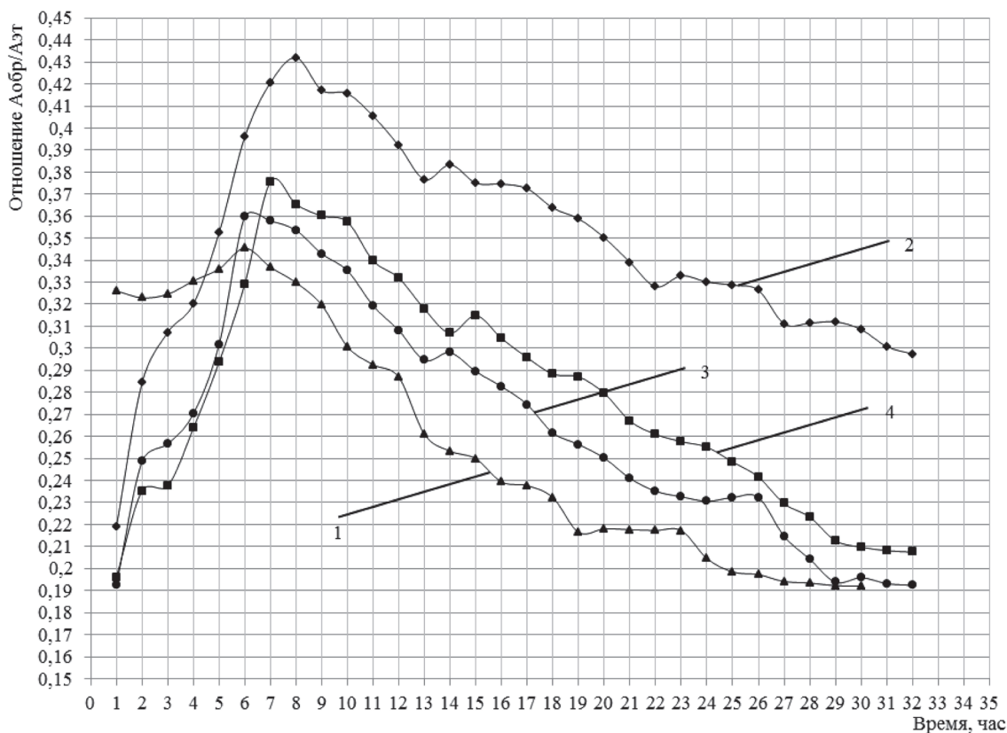
Рис. 4. Кинетика активности системы отверждения БК без П-23 и в его присутствии в разной дозировке при 80 °С: 1 – без П-23, 2 – 1,1 %; 3 – 1,5 %; 4 – 1,8 %
